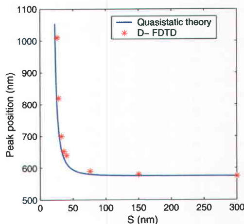
شکل ۵: تنظیم شیفت قله نوسان ساختار با تغییر فاصله دو نانودیسک (S). محاسبه شده با روش D-FDTD و مقایسه شده با تئوری تقریب الکترومغناطیسی شبه‌ساکن.
