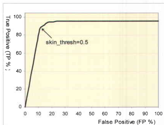
شکل ۵- نمودار ROC سیستم بر اساس مقادیر مختلف skin\_thresh
