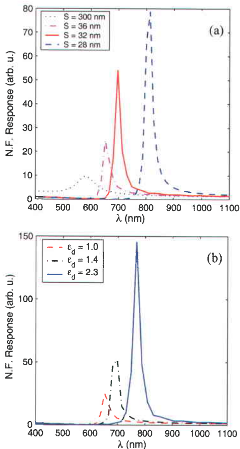
شکل ۴: پاسخ میدان نزدیک و طیف‌های شدت میدان با تغییر (a) فاصله دو نانودیسک (S) از ۳۰۰ تا ۲۸ نانومتر و (b) گذردهی الکتریکی نسبی فضای بین دو نانودیسک از ۱ تا ۲/۳، محاسبه شده با روش D-FDTD
