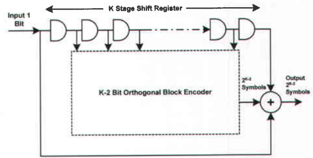
شکل ۱. ساختار اندکد super-orthogonal
